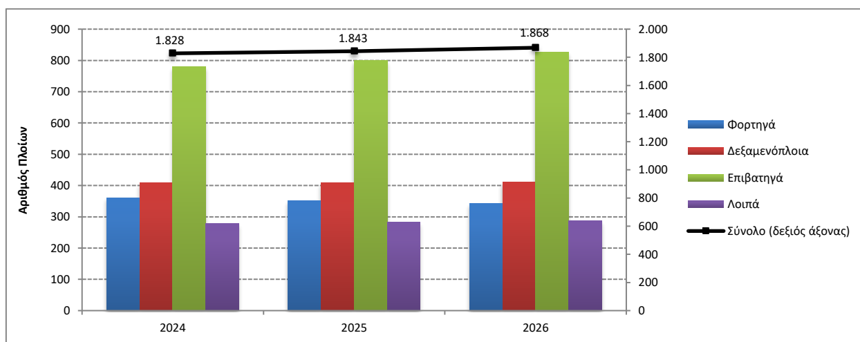
Γράφημα 2α: Δύναμη των ελληνικών εμπορικών πλοίων 100 ΚΟΧ και άνω, κατά κατηγορίες πλοίων Ιούλιος 2024 – 2026
