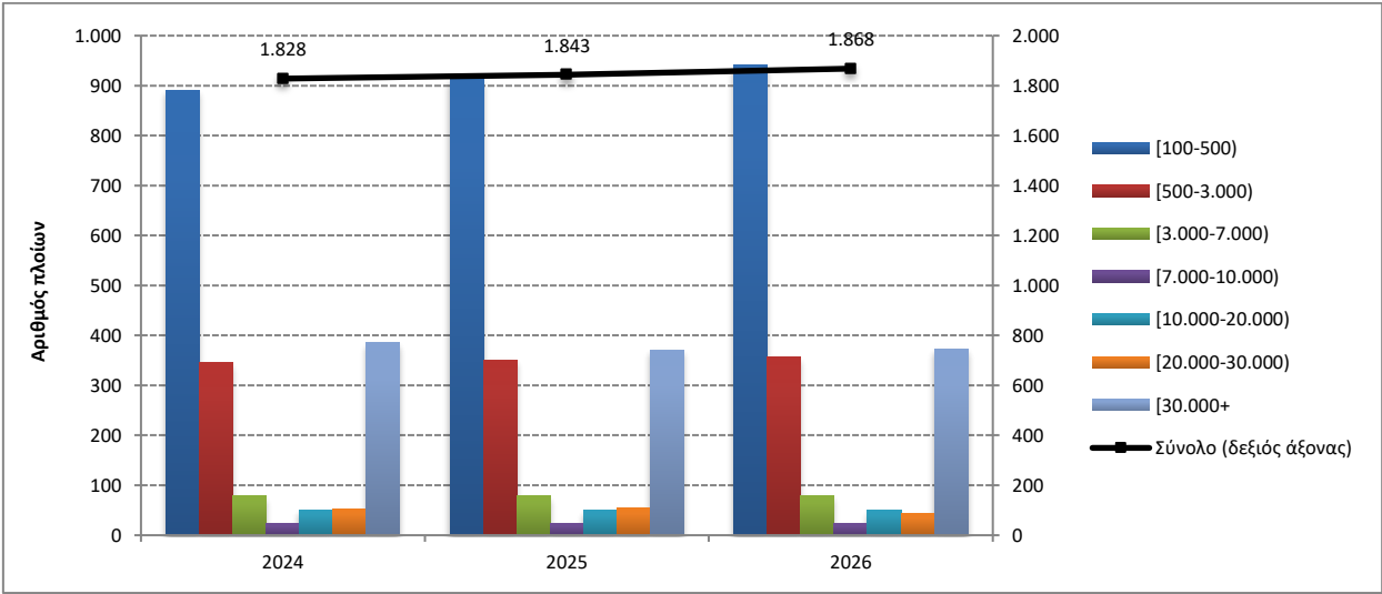
Γράφημα 3: Κατανομή των ελληνικών εμπορικών πλοίων 100 ΚΟΧ και άνω, κλιμάκια ολικής χωρητικότητας, Ιούλιος 2024 – 2026
