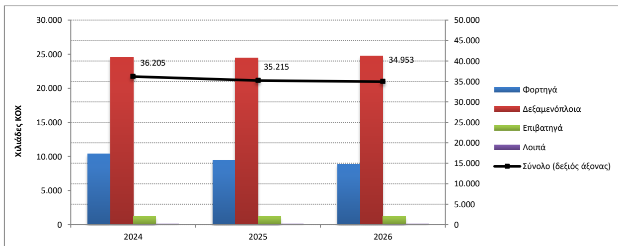
Γράφημα 2β: Χωρητικότητα των ελληνικών εμπορικών πλοίων 100 ΚΟΧ και άνω, κατά κατηγορίες πλοίων, Ιούλιος 2024 – 2026
